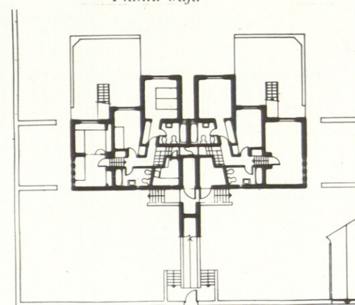
Planta alta
