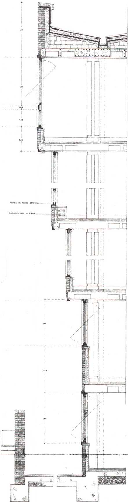
Sección constructiva.
