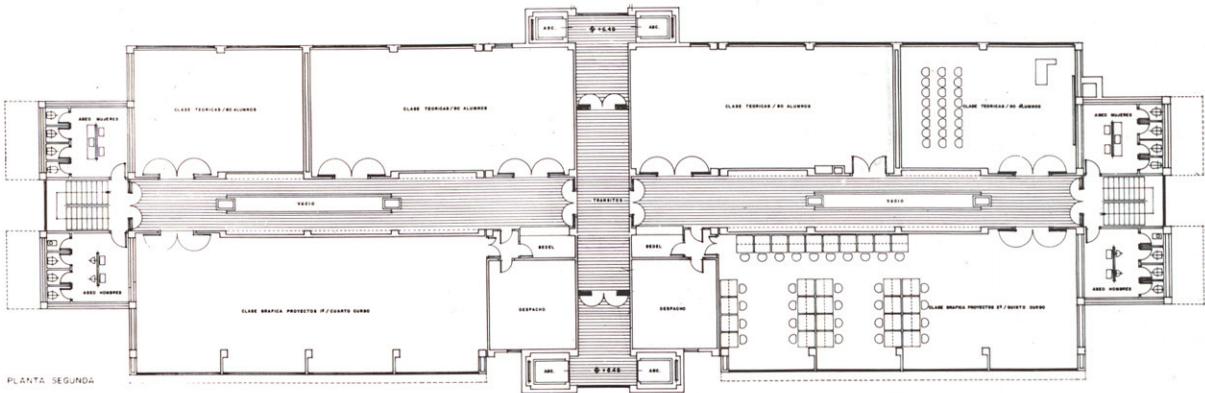
Planta segunda.
