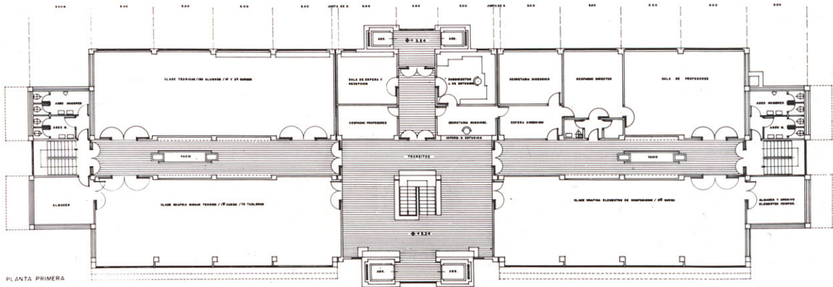
Planta primera.
