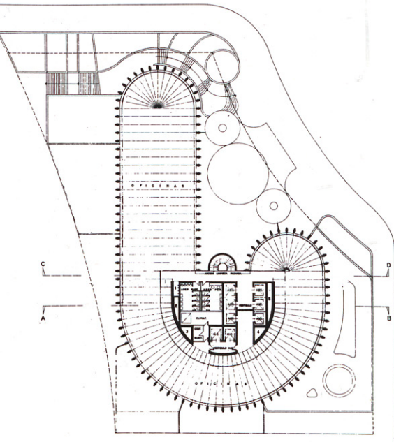
Proyecto ganador para una torre de oficinas en Azca, de Miguel de Oriol e Ibarra. Arriba, Planta Tipo y a la derecha, Alzado Sur.
