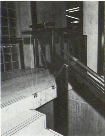
En esta página, detalles constructivos del lucernario y frentes de pavés, y vistas de la escalera.
