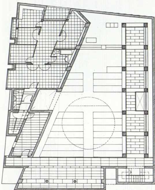
De arriba a abajo, planta de tribuna y planta de nave.
