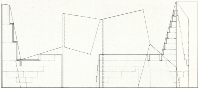
Alzado BB.
