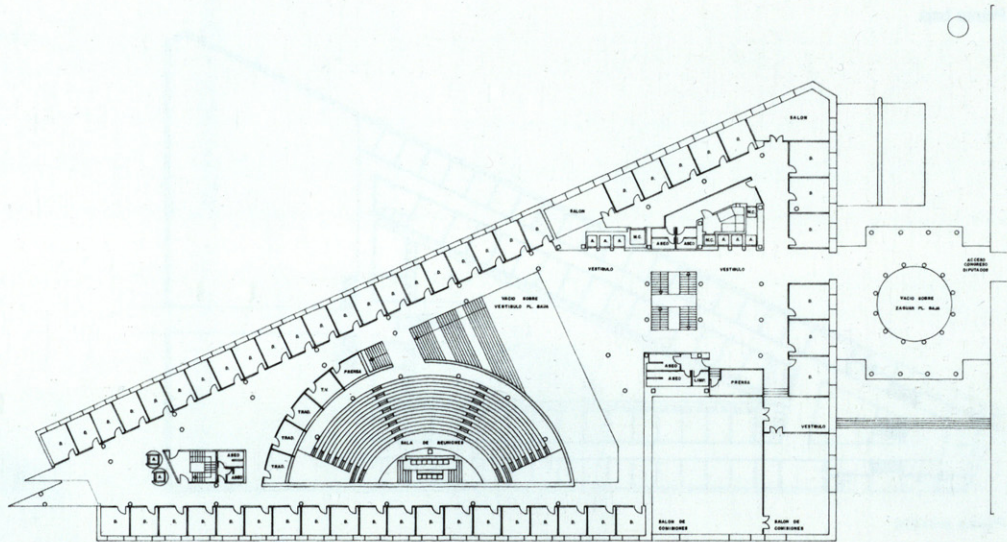
Planta primera
