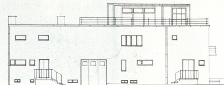
Alzado a calle.
