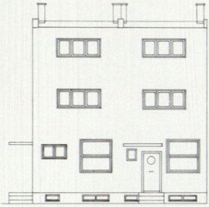
Alzado a la calle.
