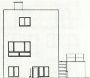
Alzado al jardín.
