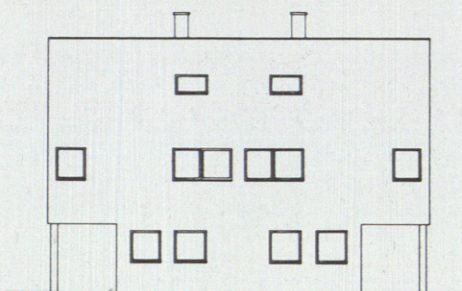
Alzado a la calle.
