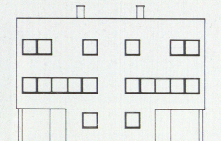
Alzado al jardín.
