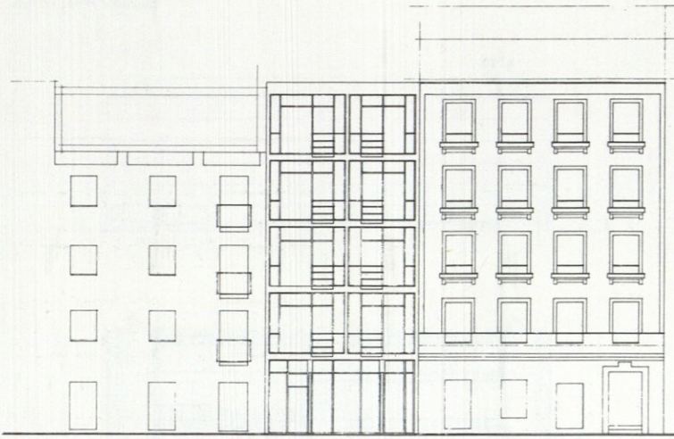
35. Alzado.
