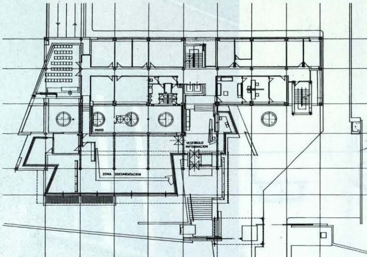
Planta primera
