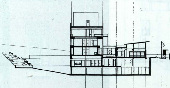
Sección transversal
