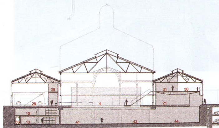
SECCIÓN NAVES LATERALES.
