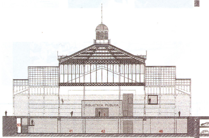
SECCIÓN PASAJE PÚBLICO.
