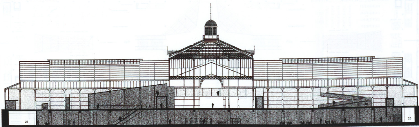
SECCIÓN VESTÍBULO.
