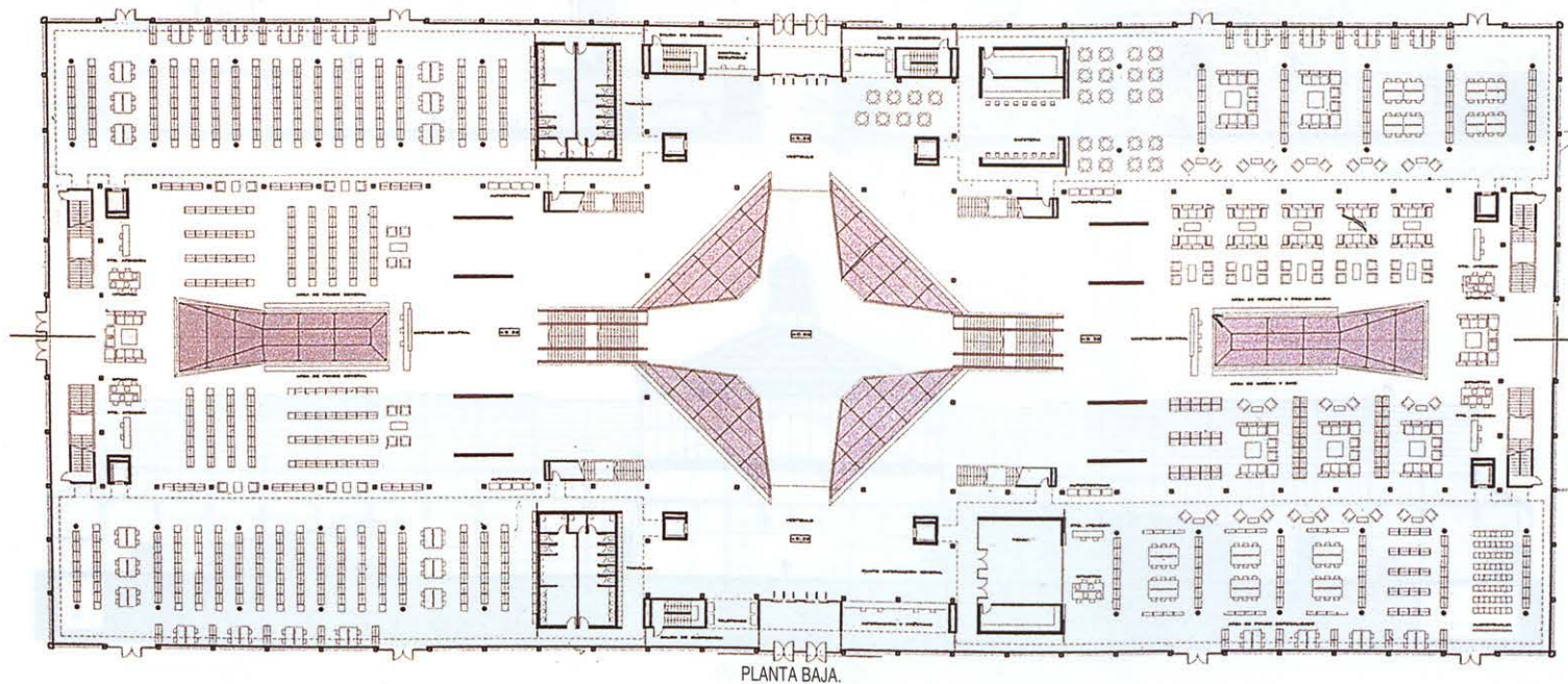
PLANTA BAJA.
