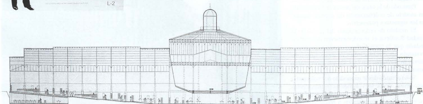
SECCIÓN LONGITUDINAL.
