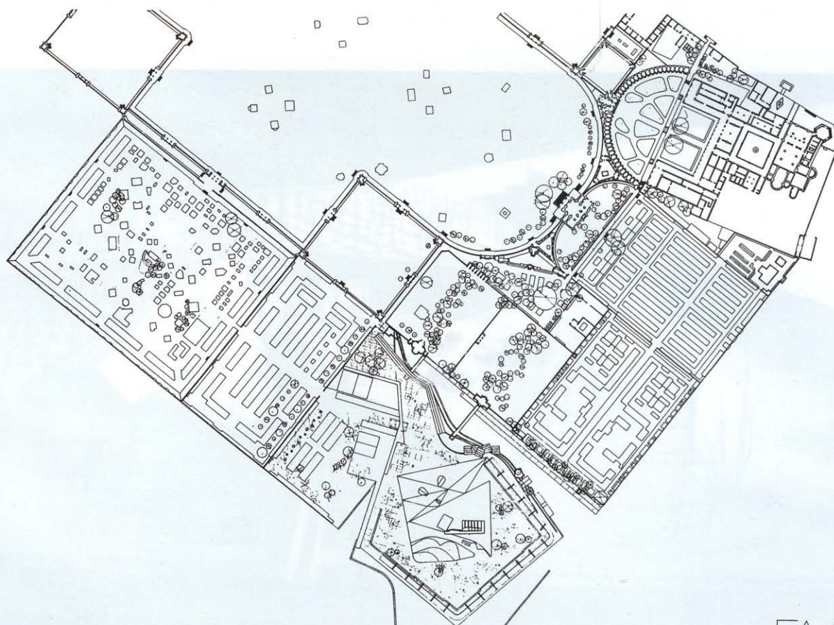
AMPLIAMENTO DEL Cimitero di SAN MICHELE IN VOLTA PLANIMETRIA GENERALE 1/1500 FAVE1
