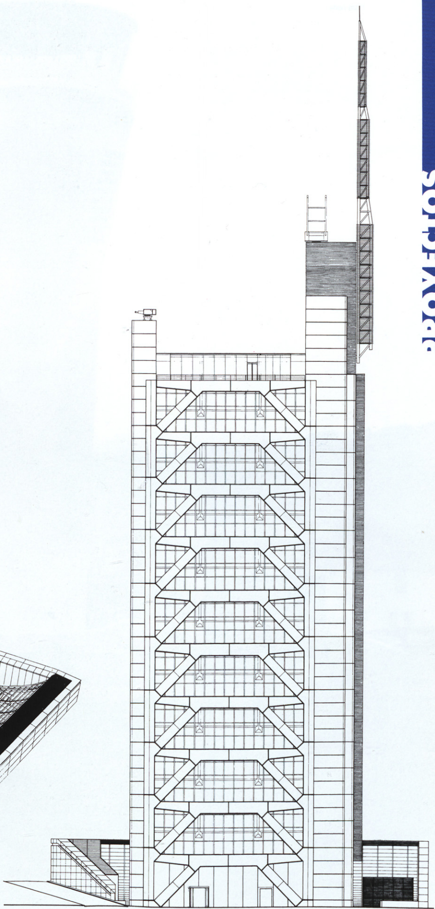
Alzado sur.
