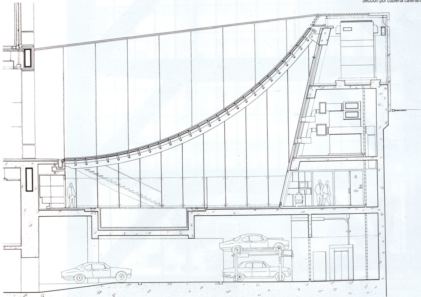
Sección por cubierta catenaria.
