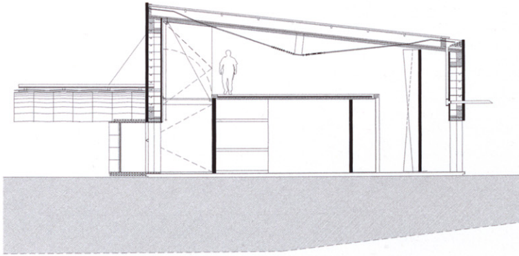
SECCIÓN TRANSVERSAL. CROSS SECTION
