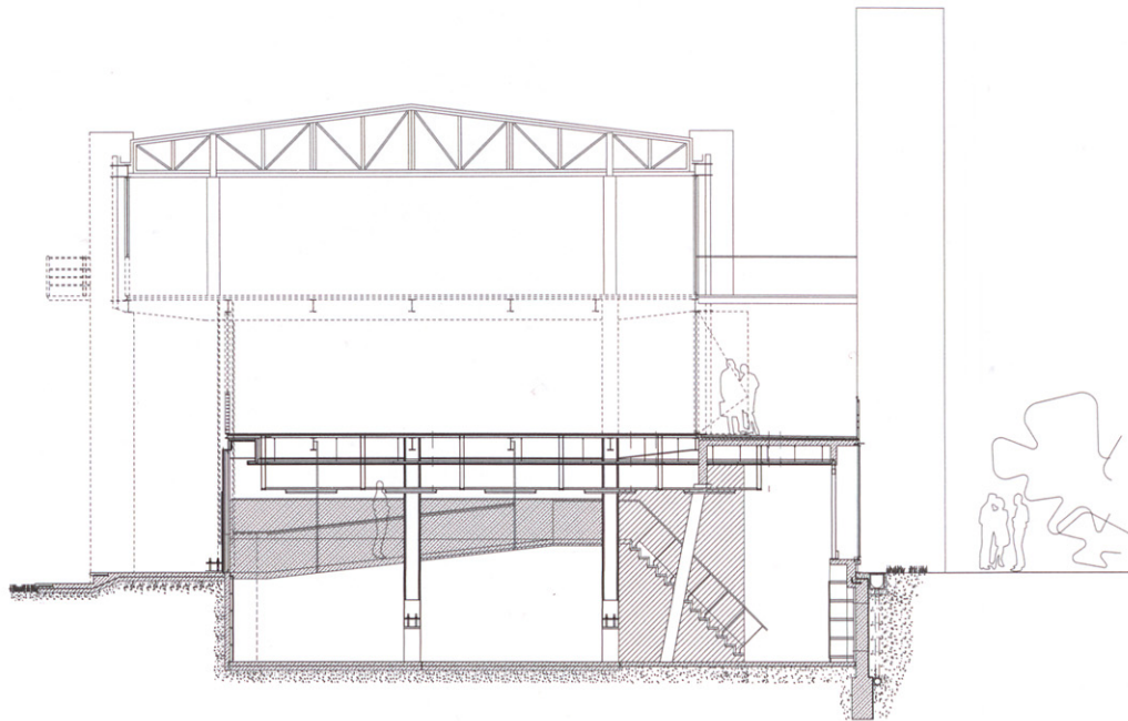
SECCIÓN TRANSVERSAL POR EL TALLER. CROSS SECTION OF THE WORKSHOP.
