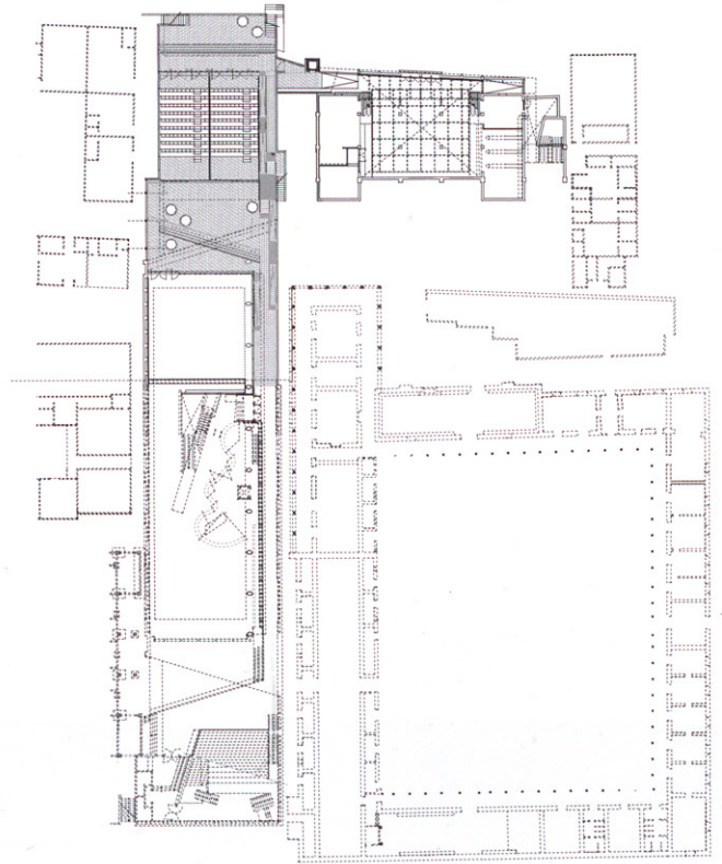
PLANTA DE ACCESO. ACCESS FLOOR
