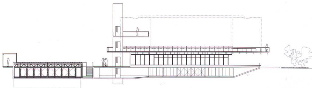
SECCIÓN TRANSVERSAL. CROSS SECTION.
