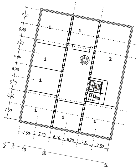
Planta Tercera
