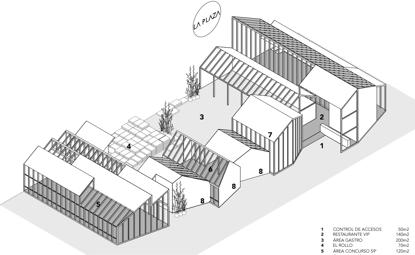
VISTA AXONOMÉTRICA
