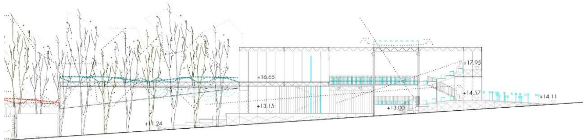
Sección longitudinal cuesta Mayano. Escala 1:300
