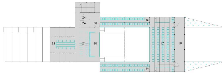
Planta primera. Escala 1:300
