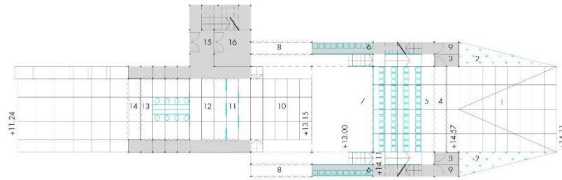
Planta calle. Escala 1:300
